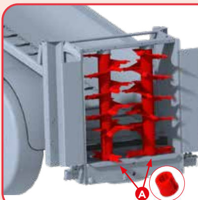
Ø 900 mm strooiwalsen met 10 mm spiralen
