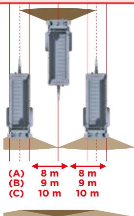
Kruisingsbreedtes (variabel afhankelijk van het gestrooide materiaal) (A) 8 m (standaard) (B) 9 m met lepelmessen (C) 10 m met strooischijven
